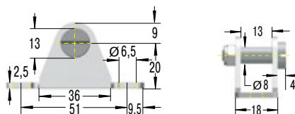
MA10-V4A Lagerschuh
