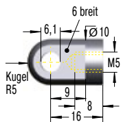
A5-VA Gelenkauge
