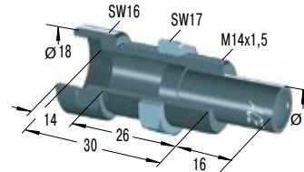
BV14SC Bolzenvorlagerung
