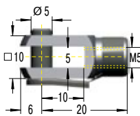
D5 Gabelkopf DIN 71752
