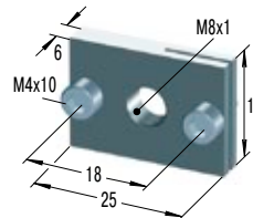
RF8 Rechteckflansch
