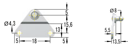
OG5-V4A Seitenbeslag
