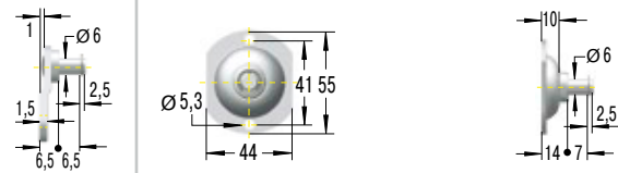
PA5 Rundbeslag
