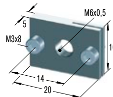
RF6 Rechteckflansch
