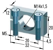
MB14 Klemmflansch
