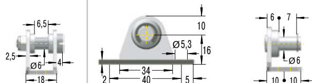
NA5-V4A Winkelbeslag
