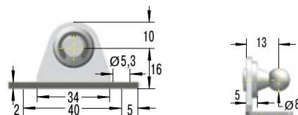
NG5-V4A Winkelbeslag
