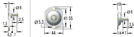
PA5-V4A Rundbeslag
