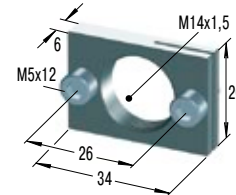
RF14 Rechteckflansch
