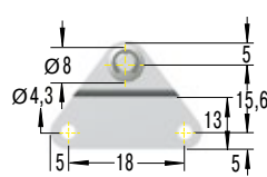
OA5 Seitenbeslag
