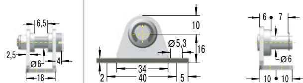
NA5 Winkelbeslag
