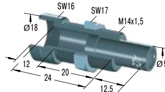
BV14 Bolzenvorlagerung
