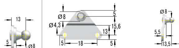
OG5 Seitenbeslag
